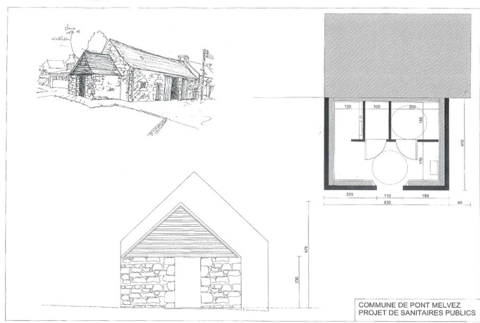
Ci-dessus: le schéma et le plan des futures toilettes publics implantées place
